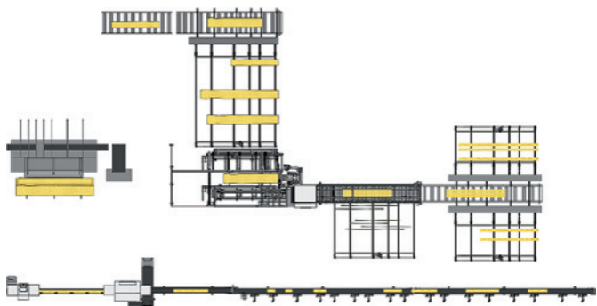
Laubholz-Zuschnittanlage mit automatischer Beschickung AB-MA_EXT, Doppelsäumer KME3, CNC-Kappanlage C14_MKL mit Sortierband, Kippenstapelung und weiteren, hochwertigen Mechanisierungskomponenten
