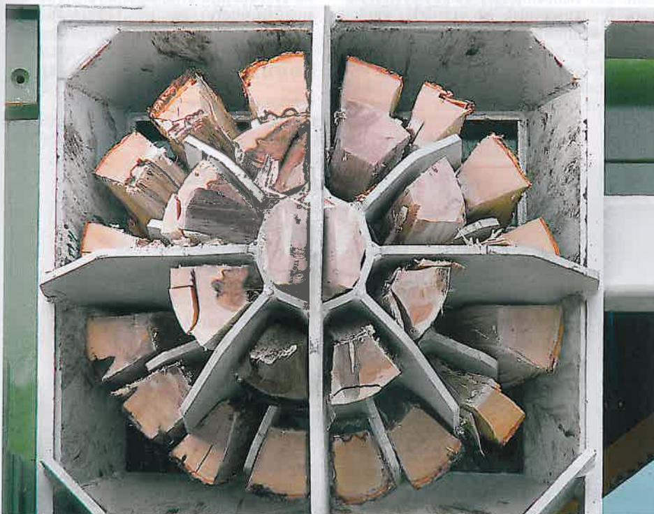
26-fach Spaltkeil für Holzsplitter-Herstellung (Pezzolato)
