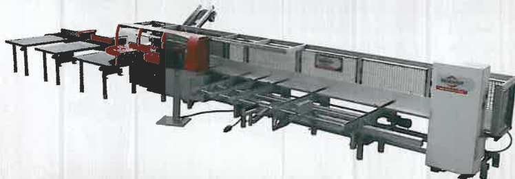
▶ Reinhardt SlimLine F, automatische Schieberkappsäge mit zusätzlicher Besäumsäge für den vollautomatischen Zuschnitt von geschlossenen Decks und Paletten
